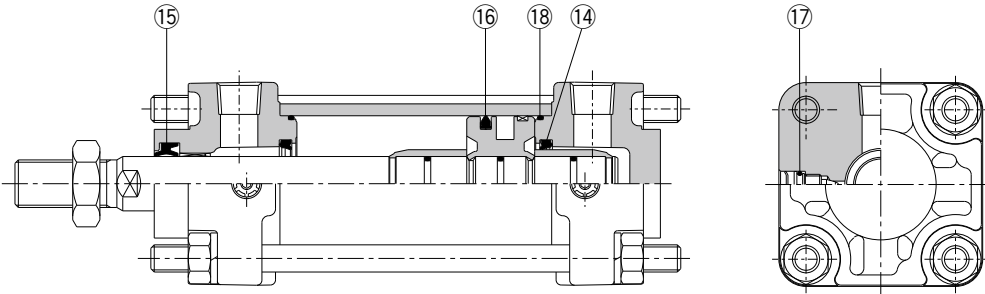
※上図はCA2シリーズの構造図です。 番号はホームページWEBカタログ CA2シリーズの構造図と同じになっています。
