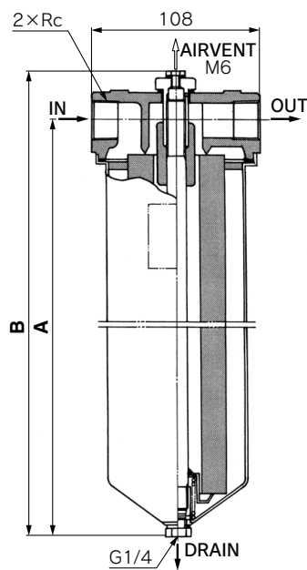
FGD□A(エレメント1本)
