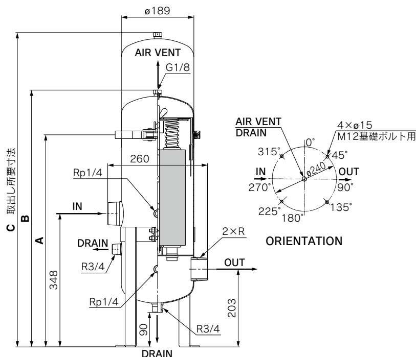
FGESタイプ(Vバンドタイプ) (mm)
