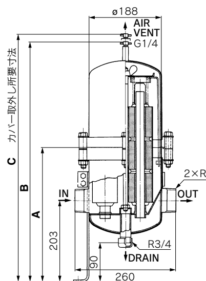
FGETタイプ(ボルト締めタイプ) (mm)
