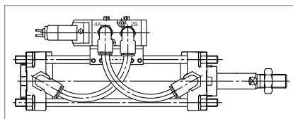
配管入れ換え / 通電引込み形
