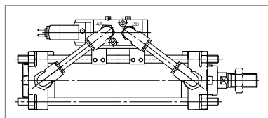
基本形 / 通電押し形
