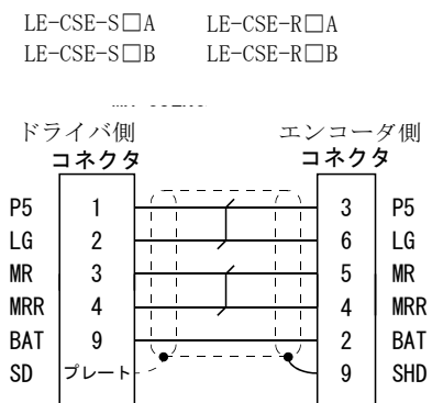
(b) ケーブル内部配線図
