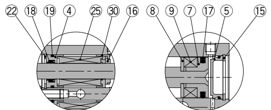
ロッドカバー部
