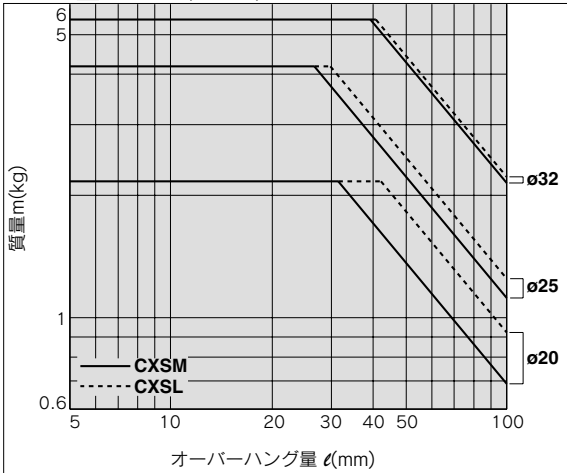
グラフ⑤ V=1000(mm/s)
