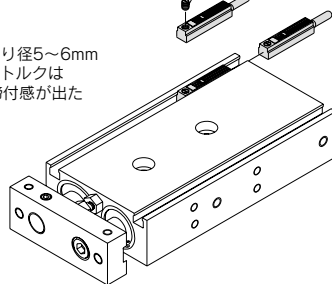
オートスイッチ取付ビス M2.5×4 \epsilon (オートスイッチに付属)
