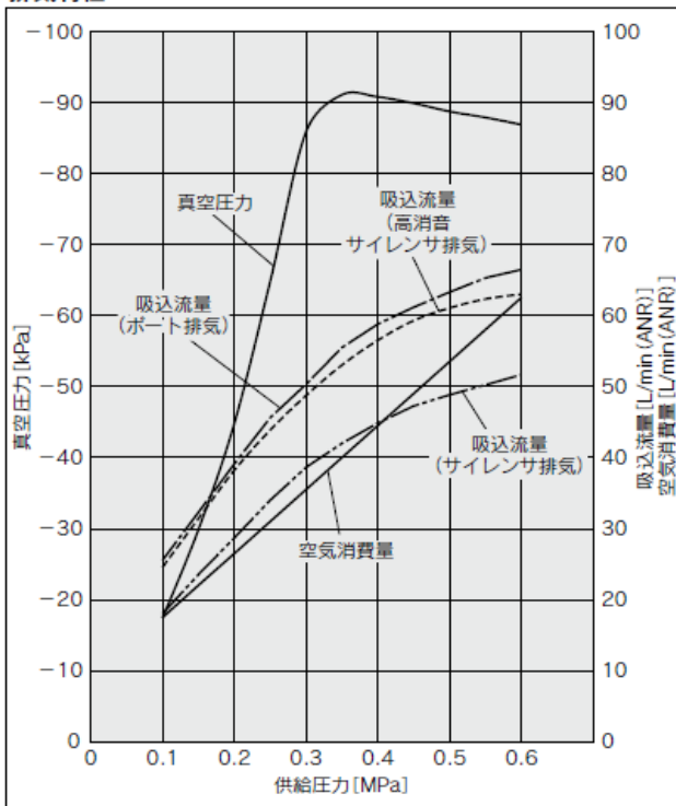
排気特性
