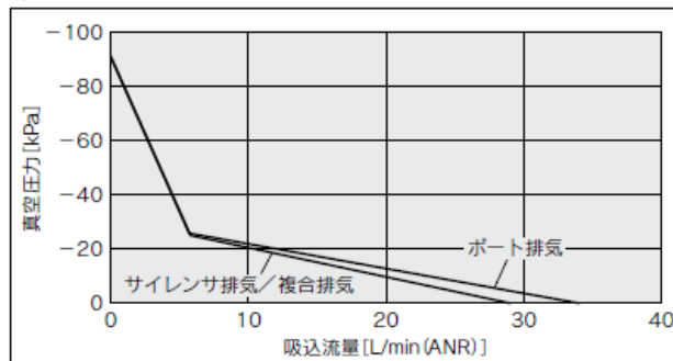
流量特性
