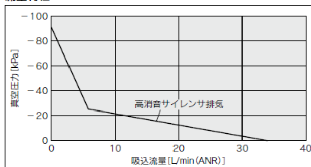
流量特性
