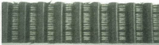
ベルト歯底摩耗（心線露出）
