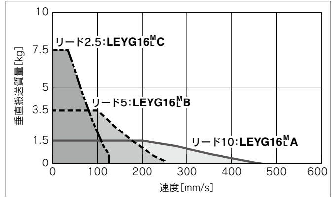
LEYG25 M □ L □ L
