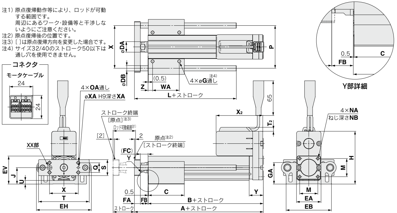
LEYG□M(すべり軸受) [mm]
