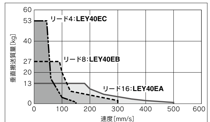
LEY40□E
