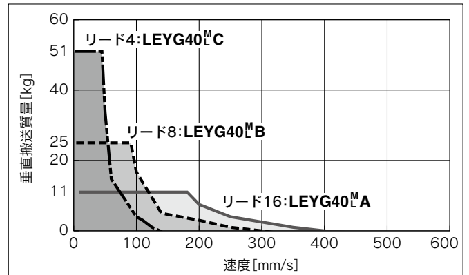
LEYG40 M □ L □ L
