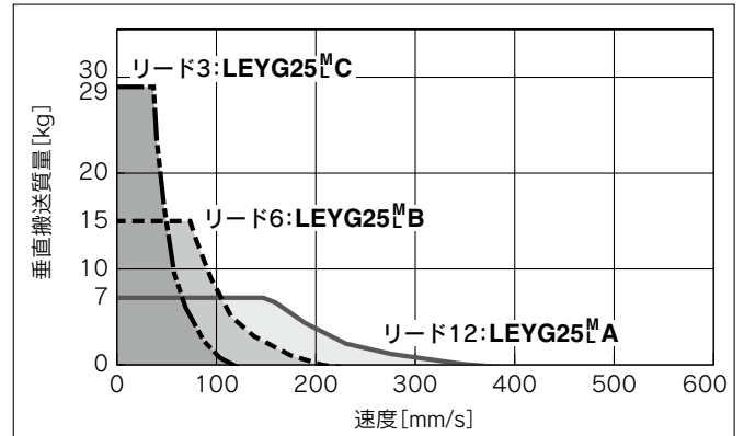
LEYG32 M □ L □ L
