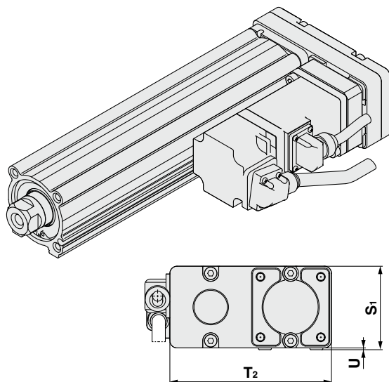
25 モータ左側折返し／LEY32L 63
