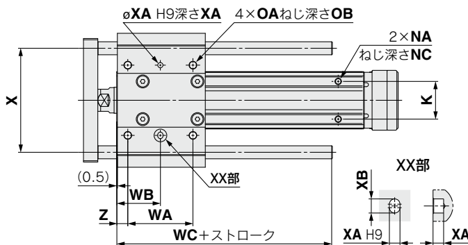
LEYG□M(すべり軸受) [mm]
