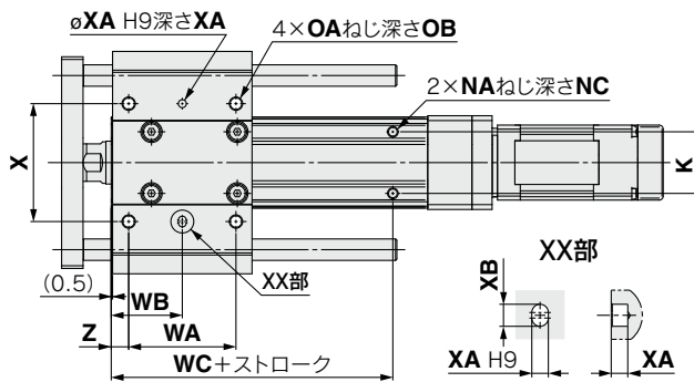
LEYG□M(すべり軸受) [mm]
