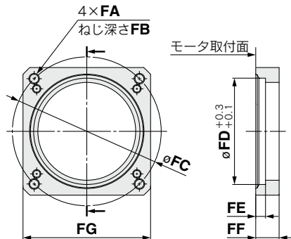
寸法表
