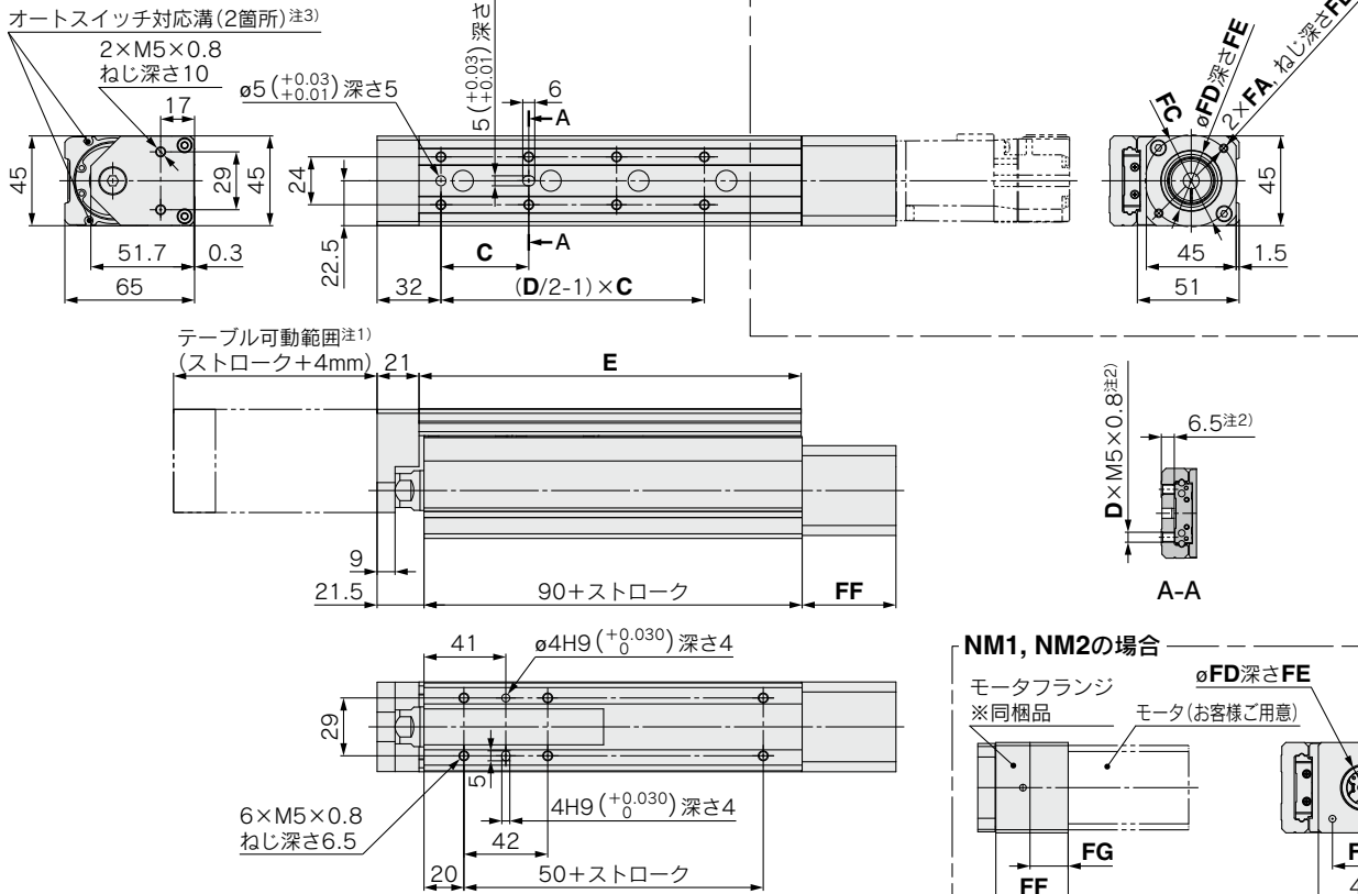
寸法表
