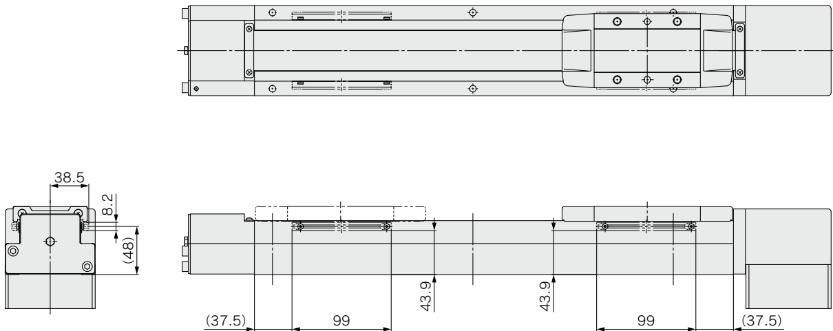
寸法表 [mm]
