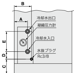
寸法表 (mm)
