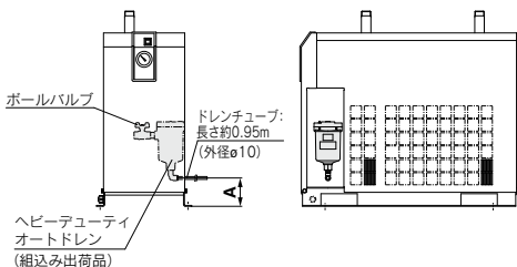
寸法表 (mm)
