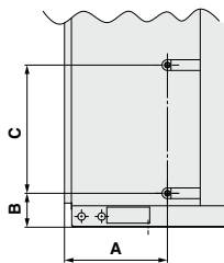
寸法表 (mm)
