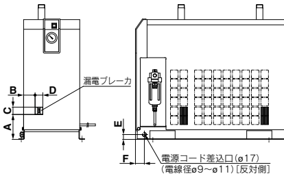
寸法表
